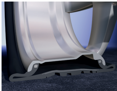
Standardirengas (tyhjentyneenä)
